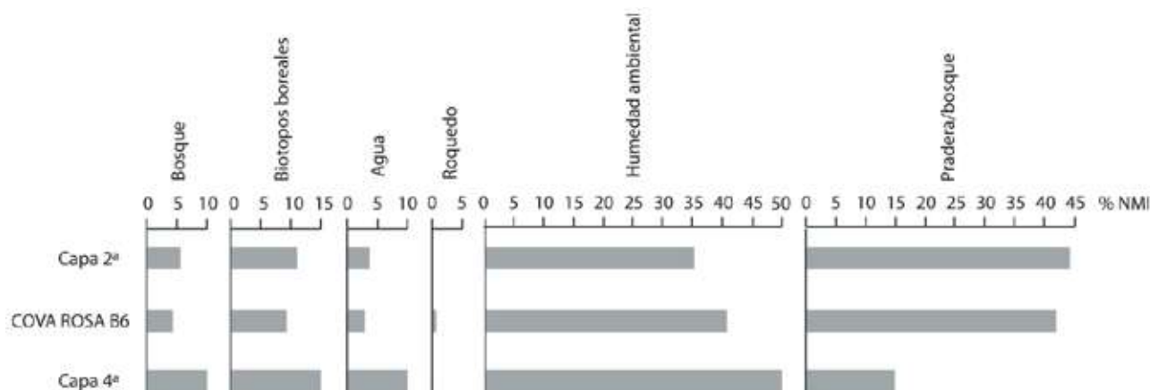
Fig. 11 – Paleoambiente inferido del estudio de los restos de microvertebrados de las Capas 2ª y 4ª (nivel I) y Cova Rosa B6 de Cova Rosa, basado en la proporción del NMI.
